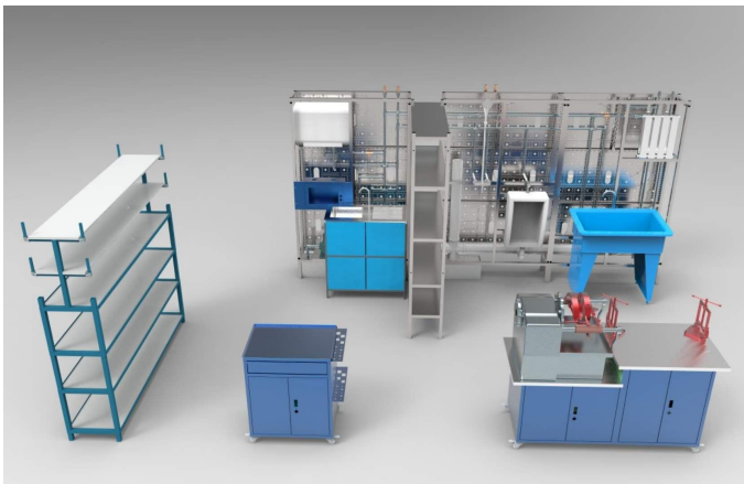
西元管道与制暖装置正面效果图
