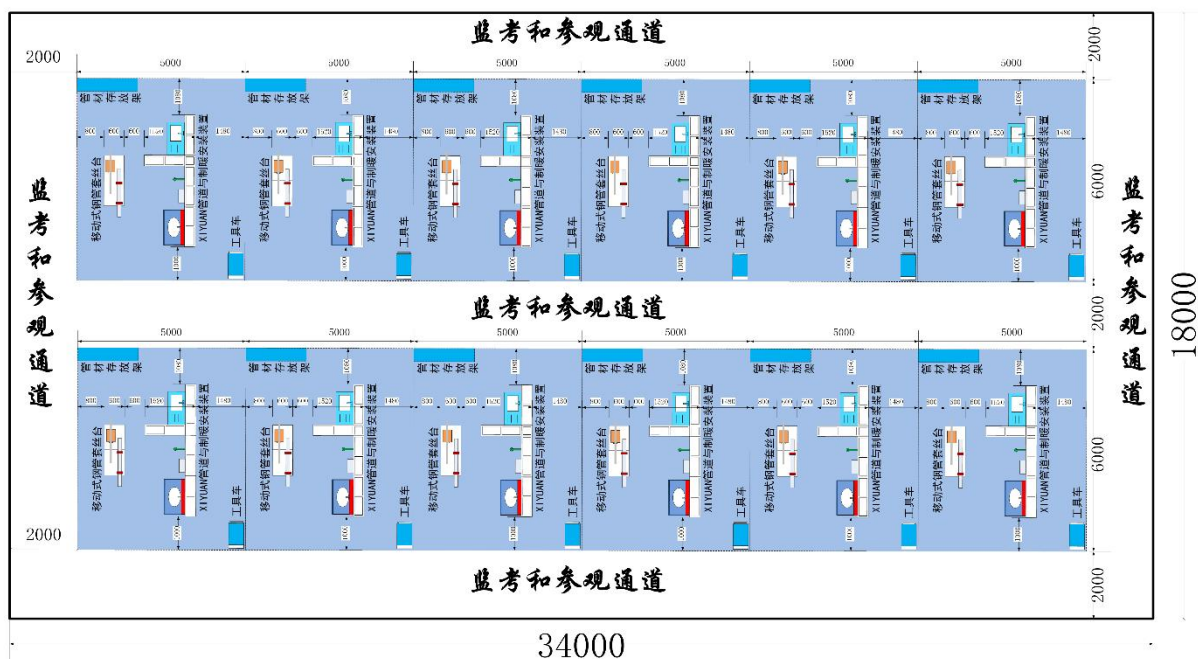
西元管道与制暖实训基地平面布局图
